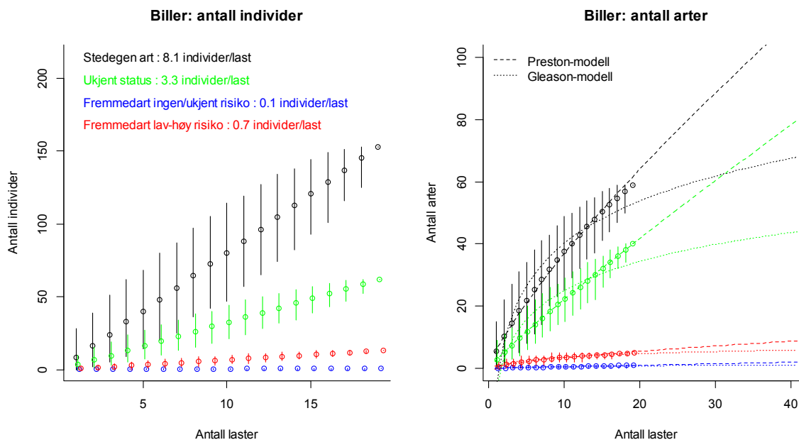
Figur 6.6. Antall individer og arter av biller som funksjon av antall laster, fordelt på stedeegne arter i Norge, arter med ukjent status og fremmede arter med ingen kjent risiko og lav-høy risiko (i henhold til siste fremmedartsliste fra Artsdatabanken; Gederaas et al. 2012). Gjennomsnitt (punkter) og 95% konfidensintervall (vertikale linjer) basert på bootstrapping (1000 gjentak). Stiplede linjer i figuren for arter (høyre) angir prediksjoner fra tilpassede modeller for akkumulasjon av arter (Y) med økende antall laster (X) med parametere a og b. Preston-modell: Y = aX^b , Gleason-modell: Y = \log(aX^b) .
