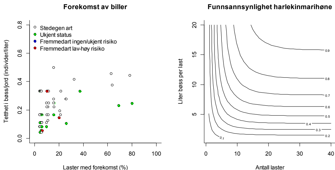
Figur 8.1. Forekomst av billearter fordelt på fremmedartsstatus (venstre) og funnsannsynlighet for harlekinmarihøne (SE – svært høy risiko) som funksjon av antall laster med potensiell forekomst og antall liter samlet per last (basert på frekvenser av harlekinmarihøne i våre data – se tekst og Vedlegg 2).
