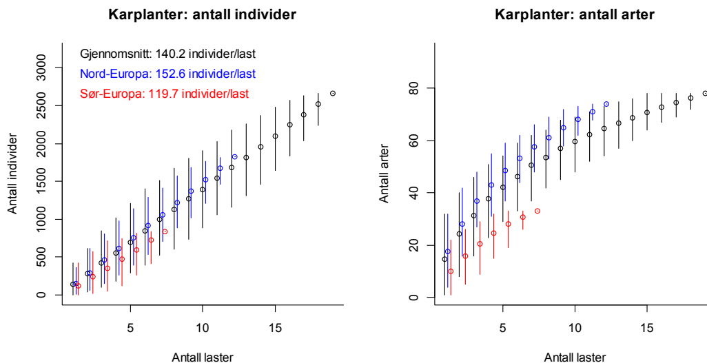
Figur 6.11. Antall individer og arter av korplanter som funksjon av antall laster, fordelt på laster fra Nord- og Sør-Europa. Gjennomsnitt (punkter) og 95% konfidensintervall (vertikale linjer) basert på bootstrapping (1000 gjentak).
